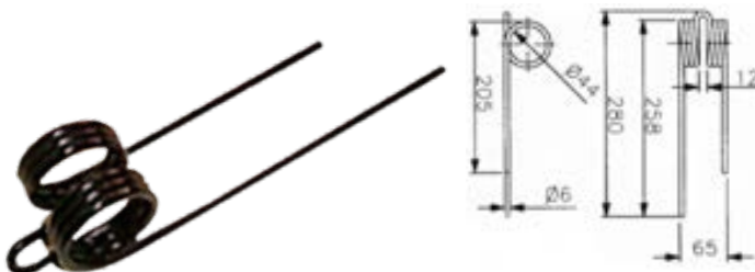
FARENDLOSE RAKE TINE FARENDLOSE 5033 5034 45.000.004
