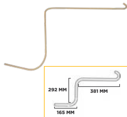
JD RAKE TINE OEM 186SE 45.160.320
