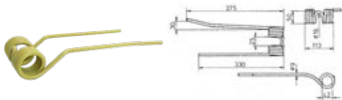
BE-TR300 NARROW RAKE TINE LH, HAYBOB 45.000.107
